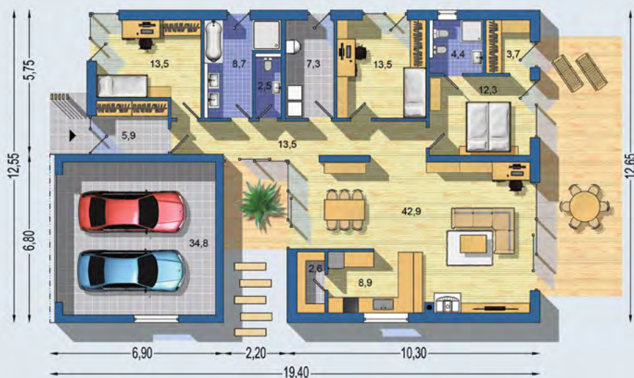
PŘÍZEMÍ [celková plocha 174.4 m 2 ]
