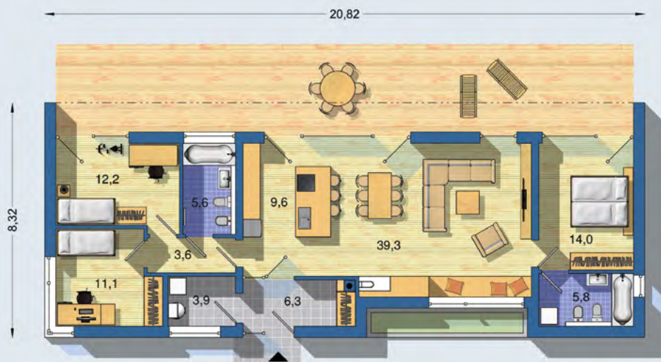
PŘÍZEMÍ [celková plocha 111.3 m 2 ]
