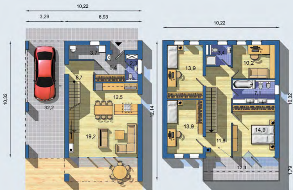
PRÍZEMÍ [celková plocha 52.7 m 2 ]
