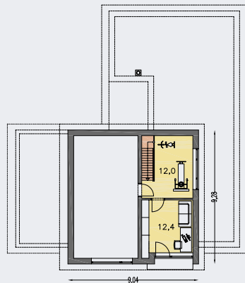
POSCHODÍ [plocha 59.9 m 2 ]
