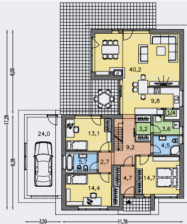
PŘÍZEMÍ [plocha 129.6 m 2 ]
