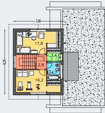
POSCHODÍ [plocha 44.9 m 2 ]
