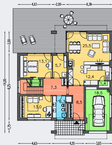
PŘÍZEMÍ [plocha 120.2 m 2 ]
