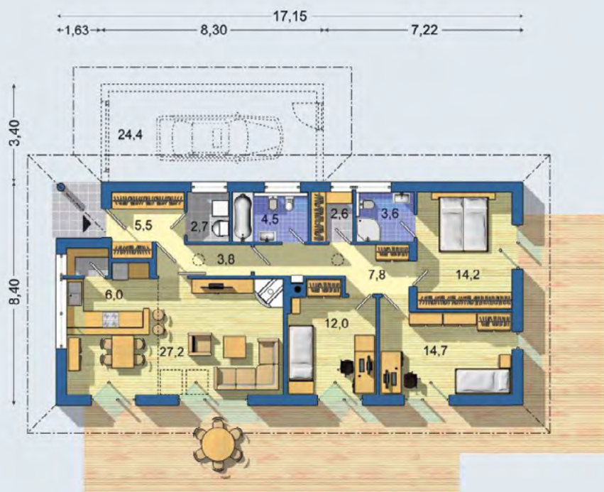
PŘÍZEMÍ [celková plocha 105.9 m 2 ]
