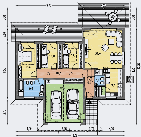
PŘÍZEMÍ [plocha 141.2 m 2 ]
