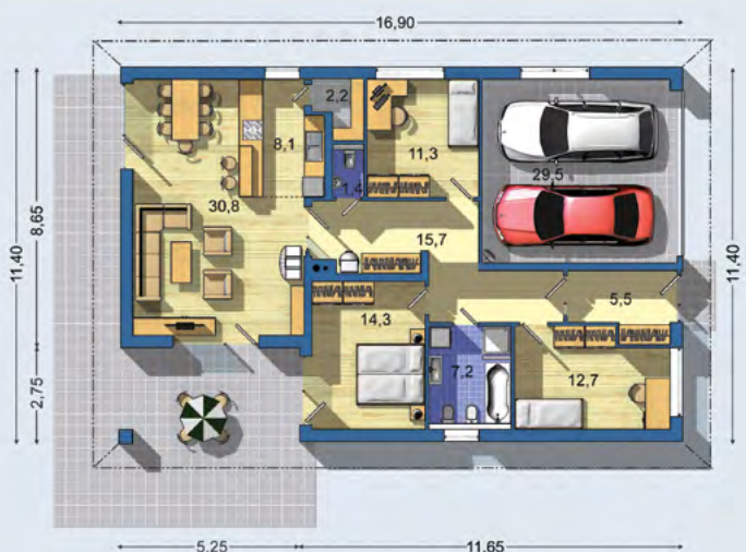
PŘÍZEMÍ [plocha 138.5 m 2 ]
