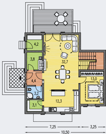
PRÍZEMÍ [plocha 84.0 m 2 ]
