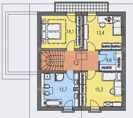
POSCHODÍ [plocha 72.8 m 2 ]
