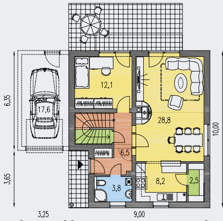
PŘÍZEMÍ [plocha 68.8 m 2 ]
