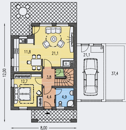
PŘÍZEMÍ [plocha 65.1 m 2 ]
