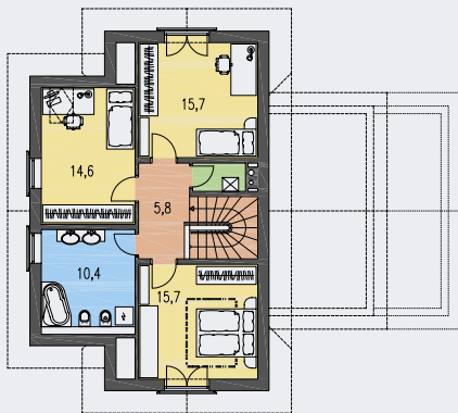
POSCHODÍ [plocha 64.0 m 2 ]
