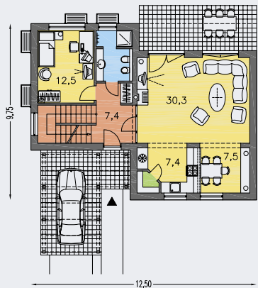
PŘÍZEMÍ [plocha 78.2 m 2 ]
