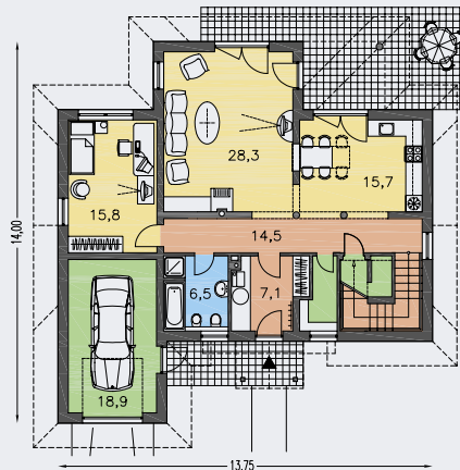
PŘÍZEMÍ [plocha 119.1 m 2 ]
