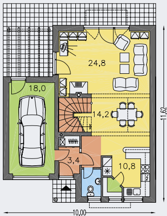
PŘÍZEMÍ [plocha 83.0 m 2 ]
