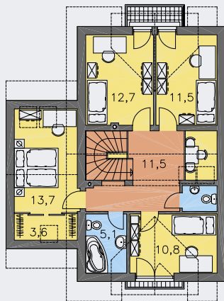
POSCHODÍ [plocha 73.4 m 2 ]
