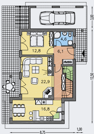
PŘÍZEMÍ [plocha 79.5 m 2 ]
