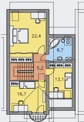
POSCHODÍ [plocha 70.6 m 2 ]
