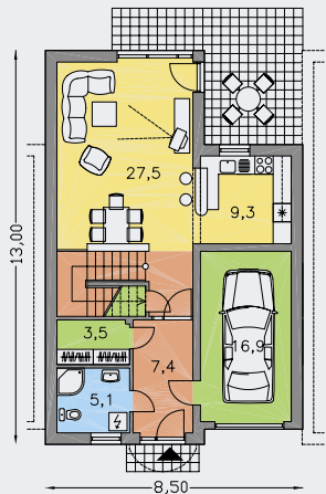
PŘÍZEMÍ [plocha 81.7 m 2 ]
