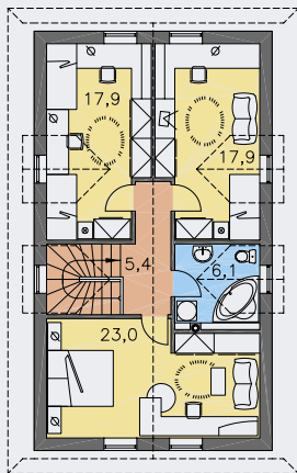
POSCHODÍ [plocha 70.2 m 2 ]
