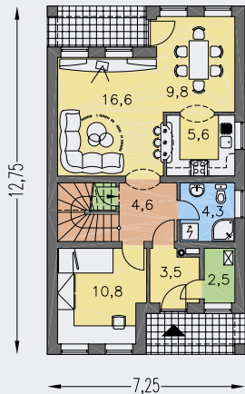
PŘÍZEMÍ [plocha 65.7 m 2 ]
