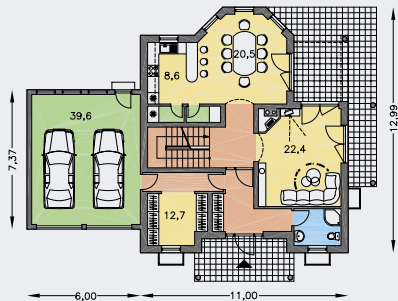
PŘÍZEMÍ [plocha 134.2 m 2 ]
