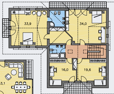
POSCHODÍ [plocha 151.8 m 2 ]
