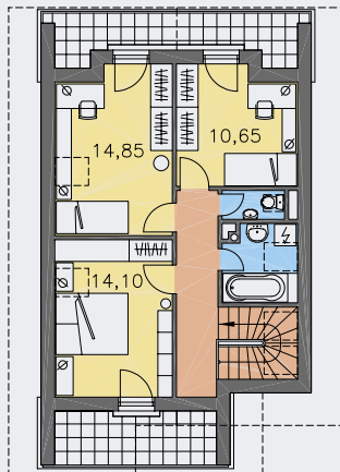
POSCHODÍ [plocha 67.6 m 2 ]
