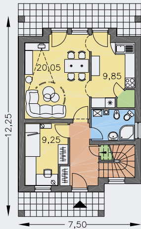
PŘÍZEMÍ [plocha 58.7 m 2 ]
