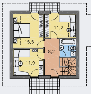
POSCHODÍ [plocha 62.4 m 2 ]
