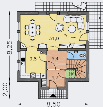
PŘÍZEMÍ [plocha 57.3 m 2 ]
