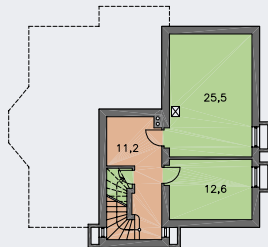
SUTERÉN [plocha 55.8 m 2 ]
