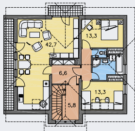
POSCHODÍ [plocha 105.2 m 2 ]
