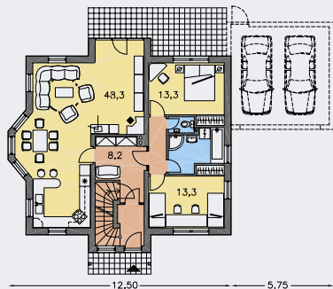
PŘÍZEMÍ [plocha 101.9 m 2 ]
