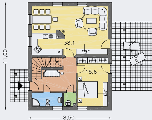
PŘÍZEMÍ [plocha 77.3 m 2 ]
