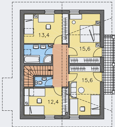
POSCHODÍ [plocha 75.9 m 2 ]
