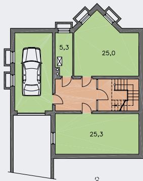
SUTERÉN [plocha 100.4 m 2 ]
