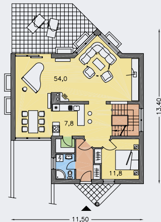
PŘÍZEMÍ [plocha 75.4 m 2 ]
