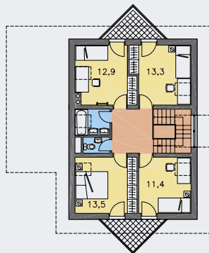
POSCHODÍ [plocha 70.8 m 2 ]
