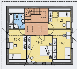
POSCHODÍ [plocha 76.9 m 2 ]
