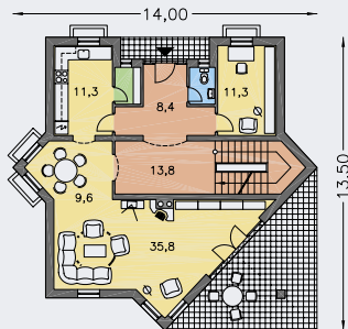
PŘÍZEMÍ [plocha 103.8 m 2 ]
