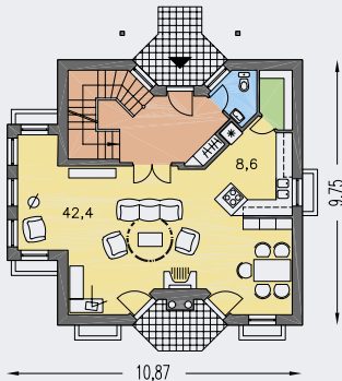
PŘÍZEMÍ [plocha 70.6 m 2 ]
