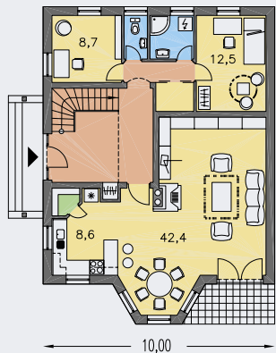
PŘÍZEMÍ [plocha 101.6 m 2 ]
