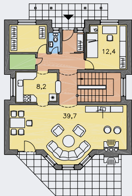
PŘÍZEMÍ [plocha 63.1 m 2 ]
