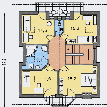
POSCHODÍ [plocha 93.4 m 2 ]
