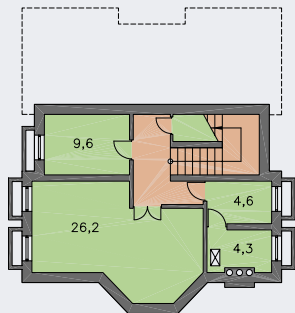
SUTERÉN [plocha 95.4 m 2 ]
