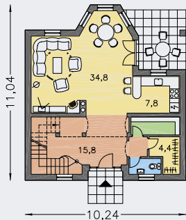
PŘÍZEMÍ [plocha 73.9 m 2 ]
