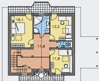
POSCHODÍ [plocha 78.9 m 2 ]
